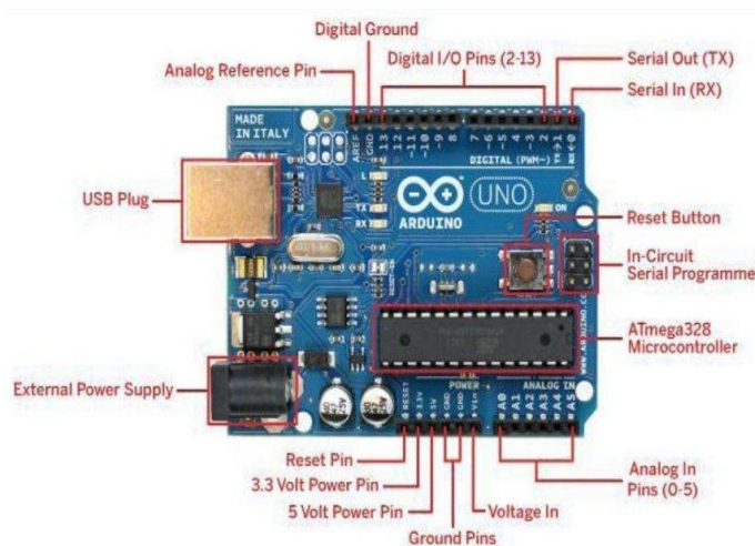
Fig. 2 Arduino UNO
